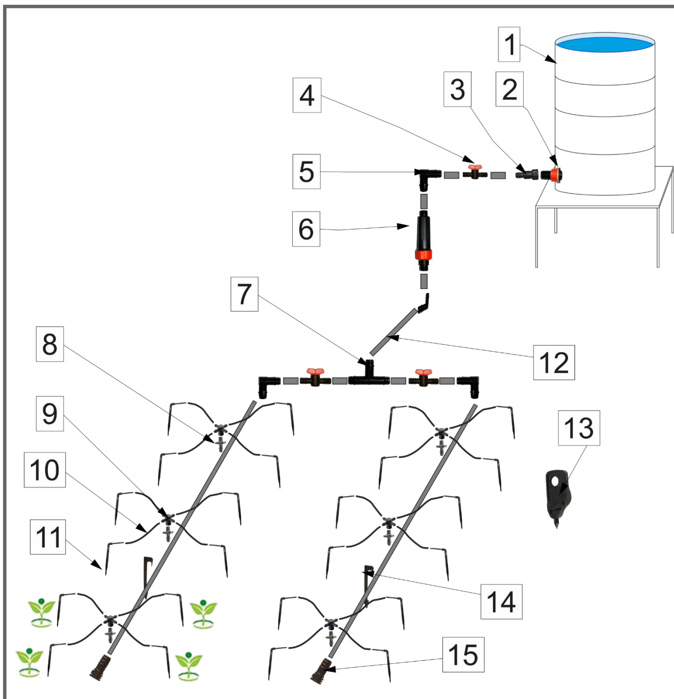
Рис.1 Схема сборки системы капельного полива
